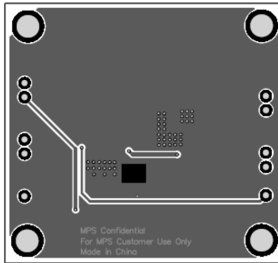
Figure 8—Bottom Layer
