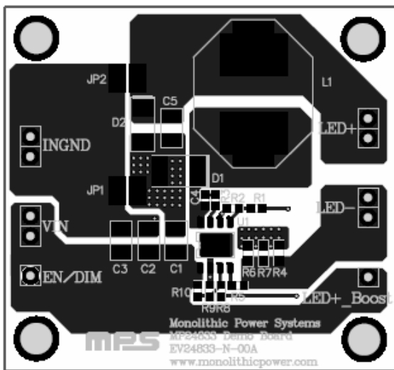
Figure 7—Top Layer
